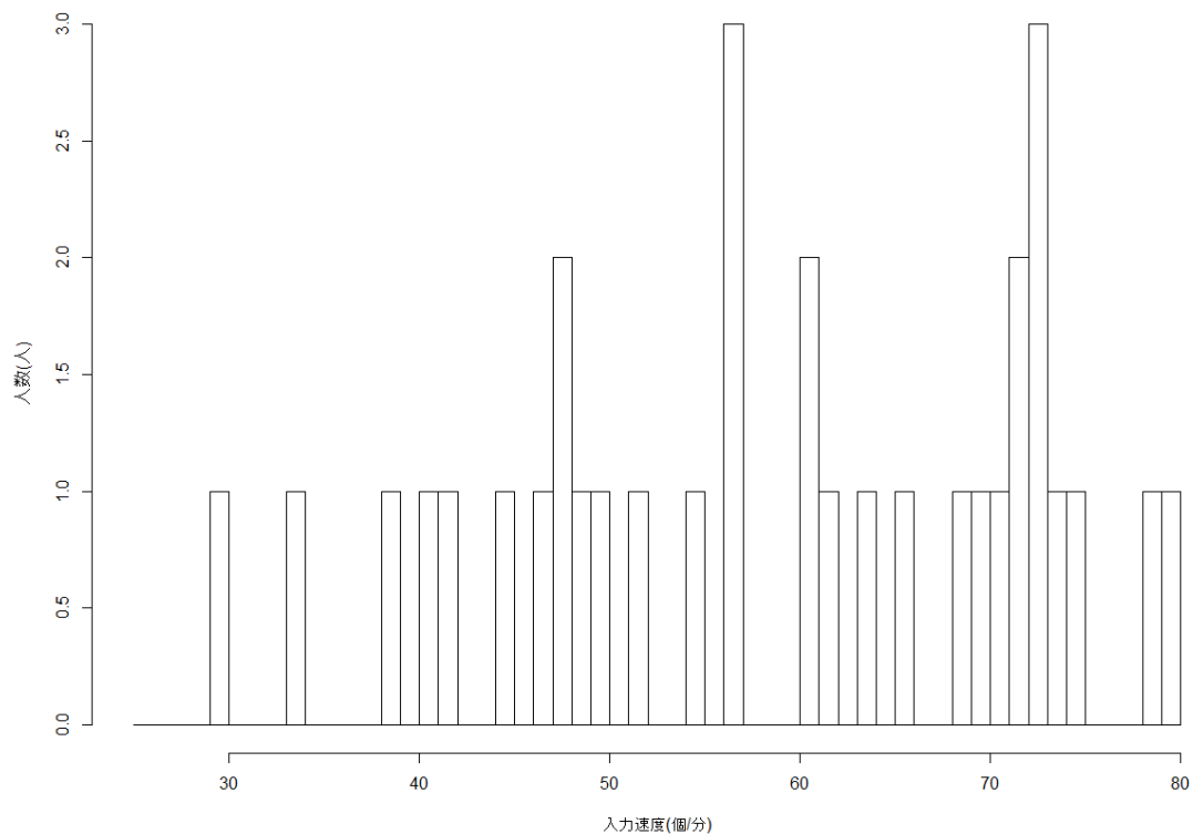
図10 速度のヒストグラム
